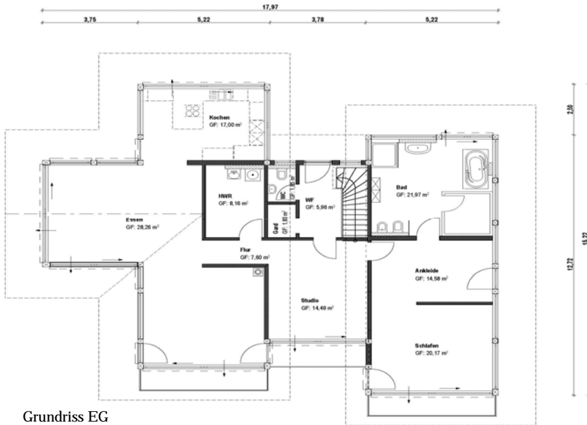
Grundriss EG
